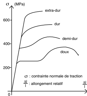
Courbe contrainte-déformation de différents aciers
